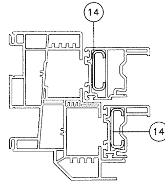
SIDE STILE
